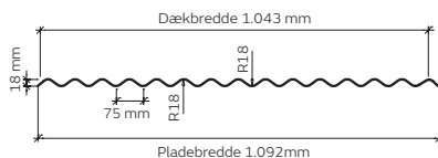
DS Sinus 18-75 (Vægprofil)
