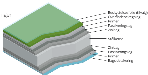
GreenCoat® materialeopbygning.
